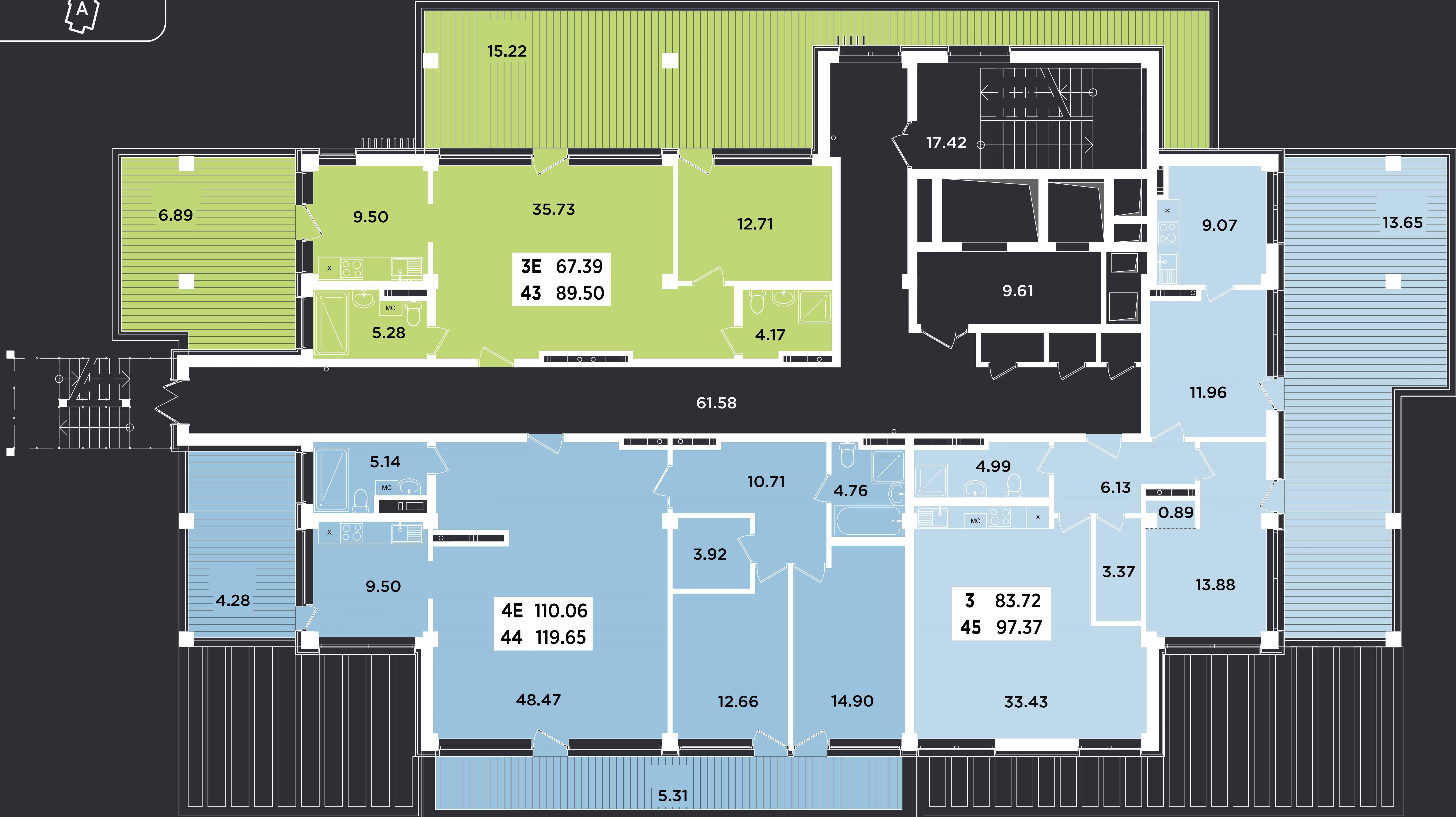
План 8 этажа 2-комнатная квартира 3-комнатная квартира
